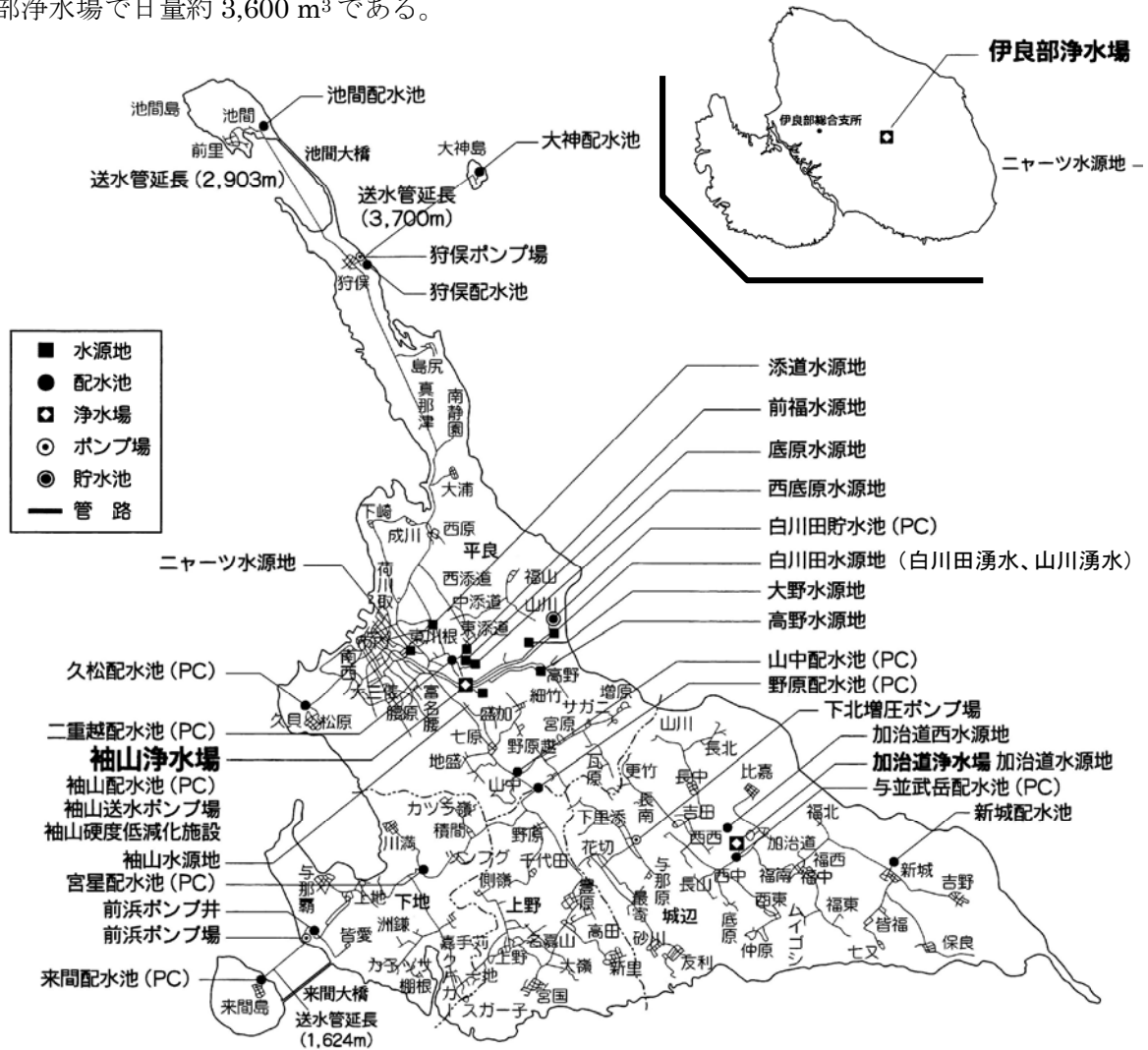
図3-1 宮古島の水道配管・施設概観図
