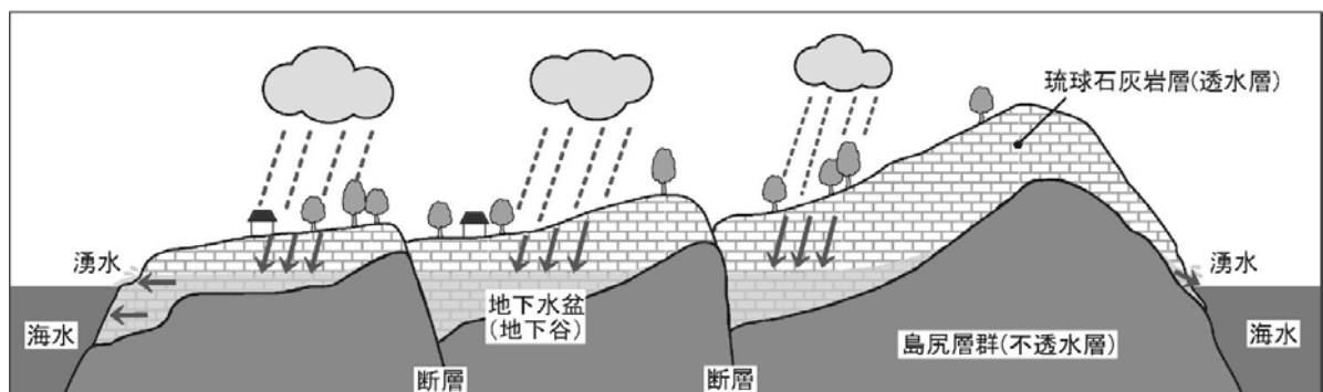
図 2-9 宮古島の模式水理地質
